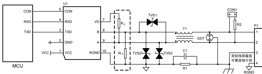
图 2 推荐应用电路图
