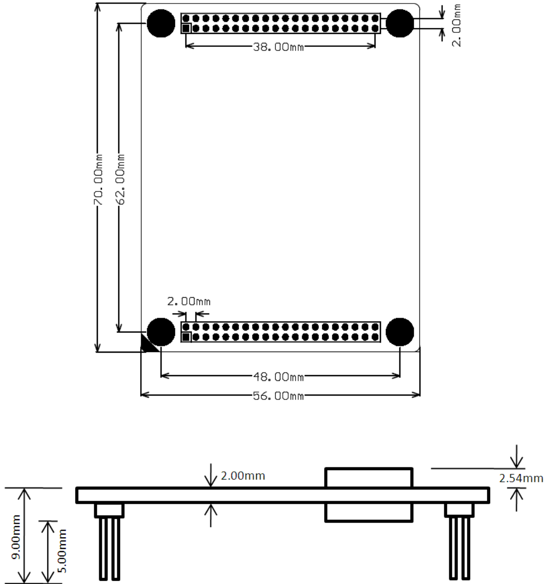
图 1.2 CANET-4E-Core 安装机械尺寸
