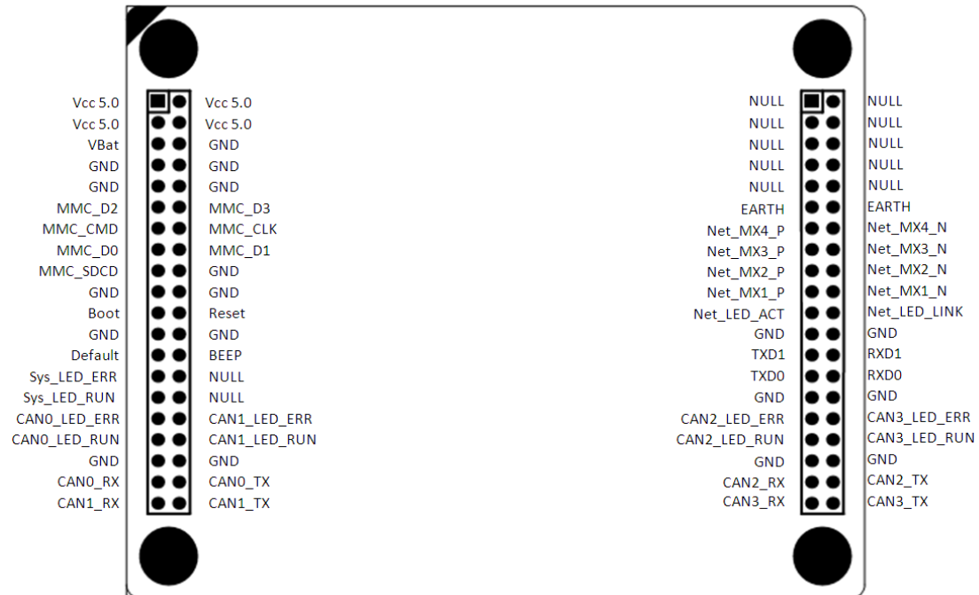
图 2.1 CANET-4E-Core 管脚定义
