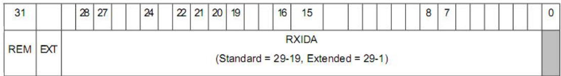
图 2.4 验收码和屏蔽码位定义
