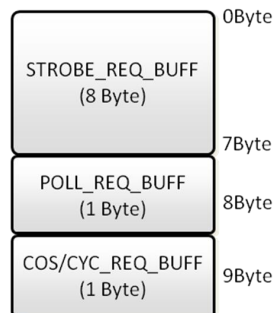
图 5.2 默认输出数据缓冲区
