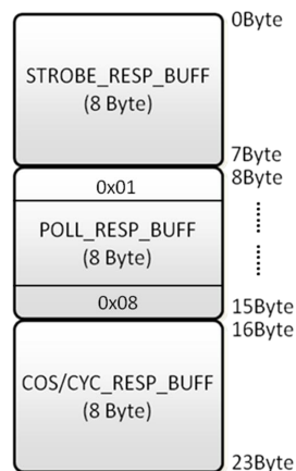
图 5.1 向轮询应答区写入输出数据
