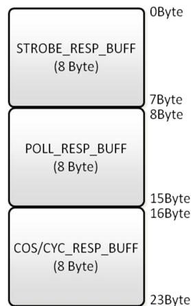
图 4.2 I/O 数据输入数据缓冲区
