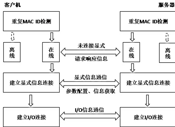
图 2.2 典型的 DeviceNet 设备连接流程
