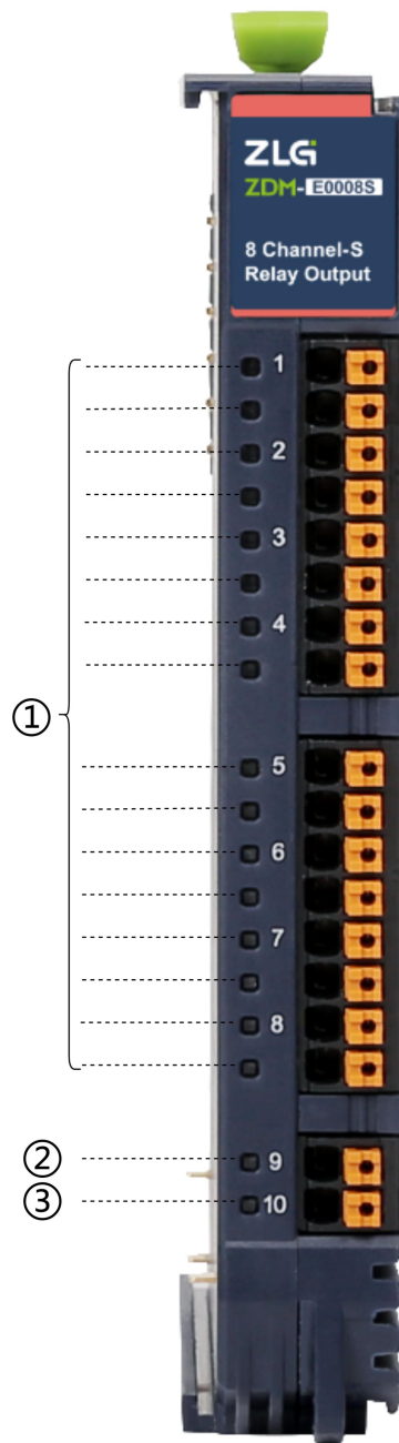
图 2.2 指示灯面板
