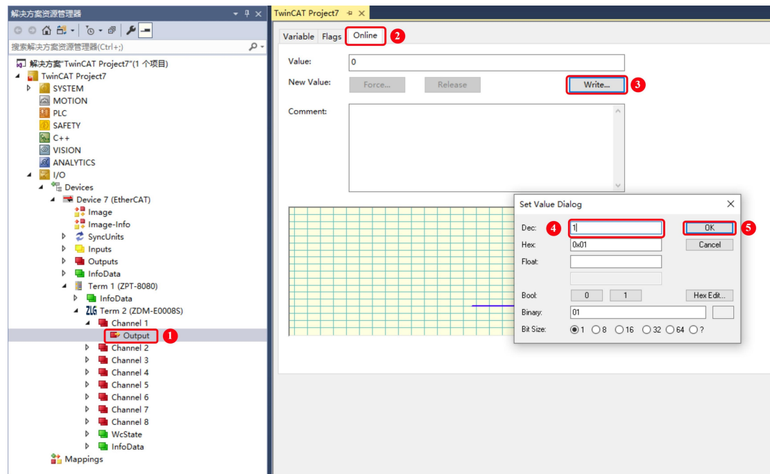
图 5.16 设置通道 1 输出有效
