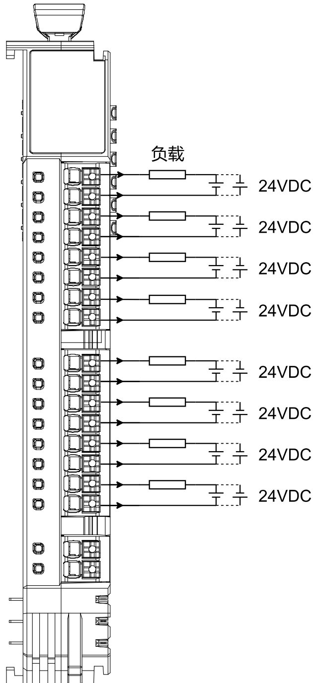
图 3.1 ZDM-E0008S 模块接线图
