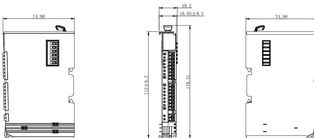
图 4.1 ZDM-E0008S 产品尺寸
