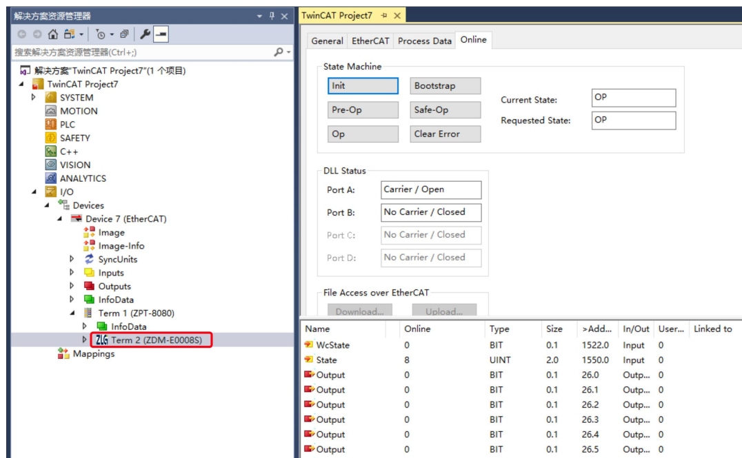
图 5.13 设备扫描成功界面
