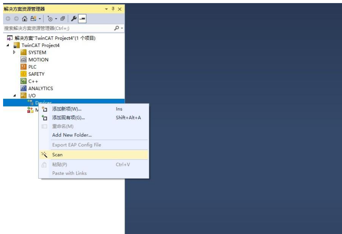
图 5.8 扫描设备
