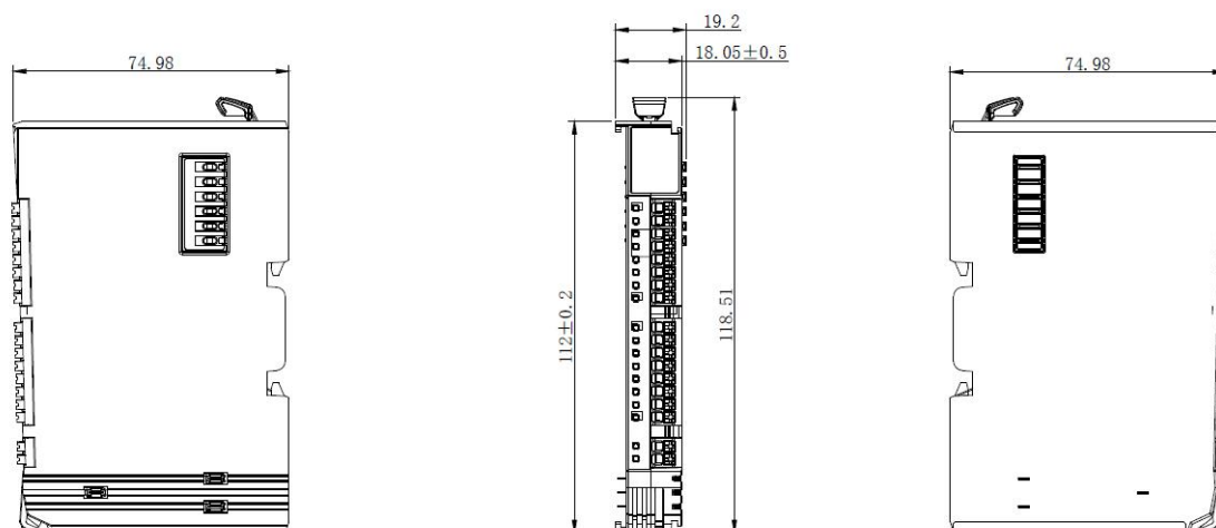
图 4.1 ZDM-E1600N 产品尺寸
