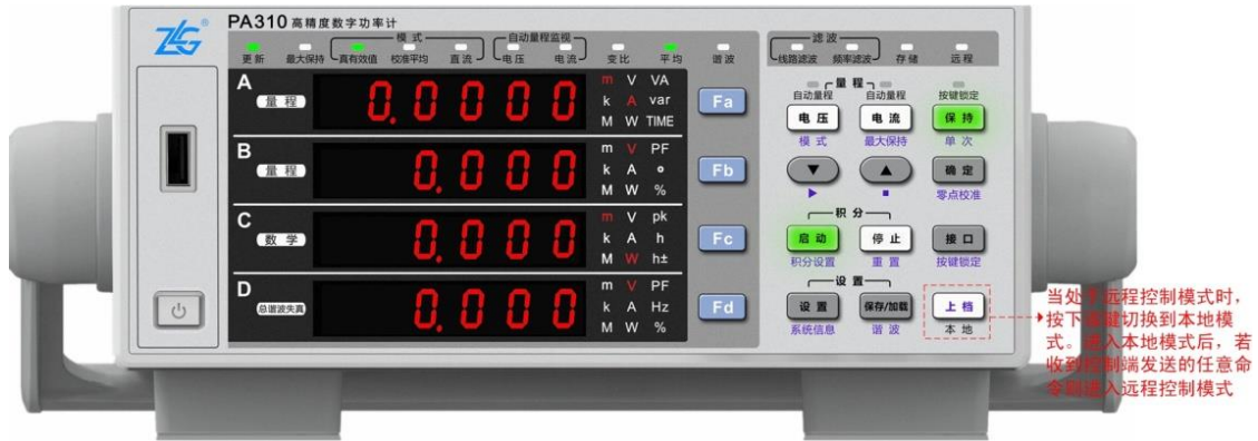
图 1.1 前面板相关按钮
