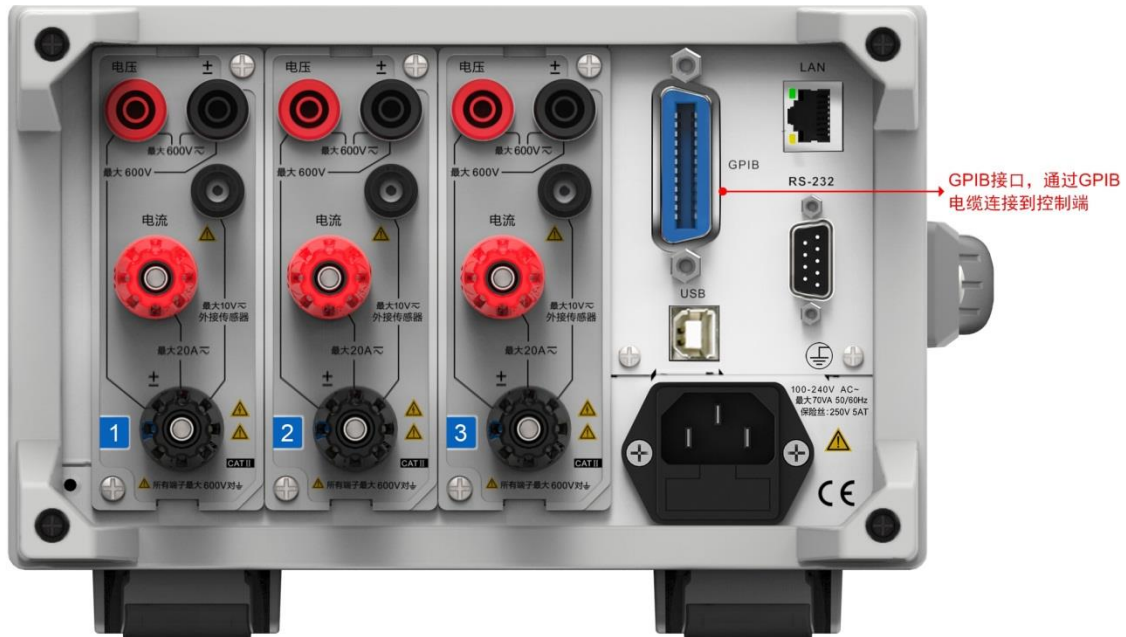
图 2.3 PA323/PA333H 型功率计 GPIB 接口
