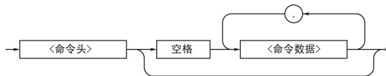
图 5.2 命令消息单元的语法
