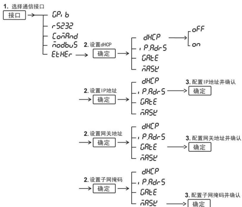
图 4.4 Ethernet 接口设置流程
