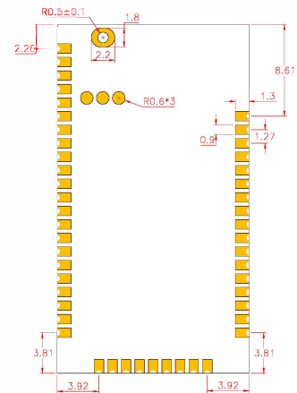
BOTTOM视图
