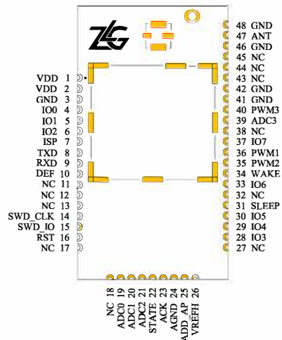
引脚分布图
